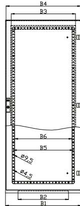
单门结构
